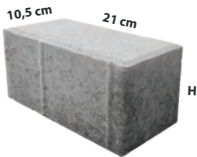
Tru Pave 21 cm x 10,5 cm Tebal 6 cm, 8 cm & 10cm 44 pcs/m2
