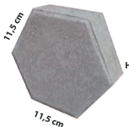
Hexagon 11,5 cm x 11,5 cm x 20 cm Tebal 6 cm & 8 cm 29 pcs/m2
