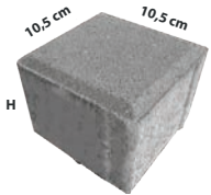
Half Pave / Kubus 10,5 cm x 10,5 cm Tebal 6 cm & 8 cm 88 pcs/m2
